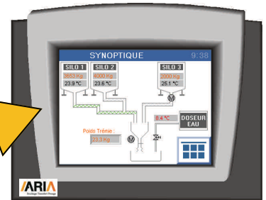
SYNOPTIQUE
